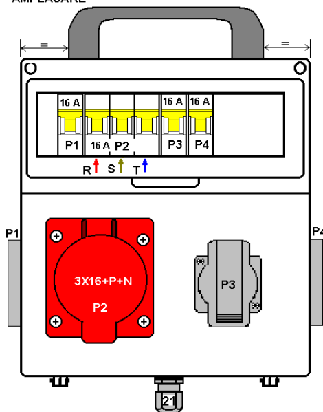
TE - SANTIER T 1x16+M3x16 A AMPLASARE
