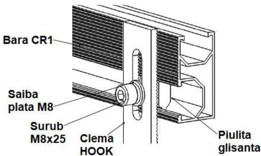
Fig. 2 - Instalare Clema HOOK pentru sistem acoperis tigla
