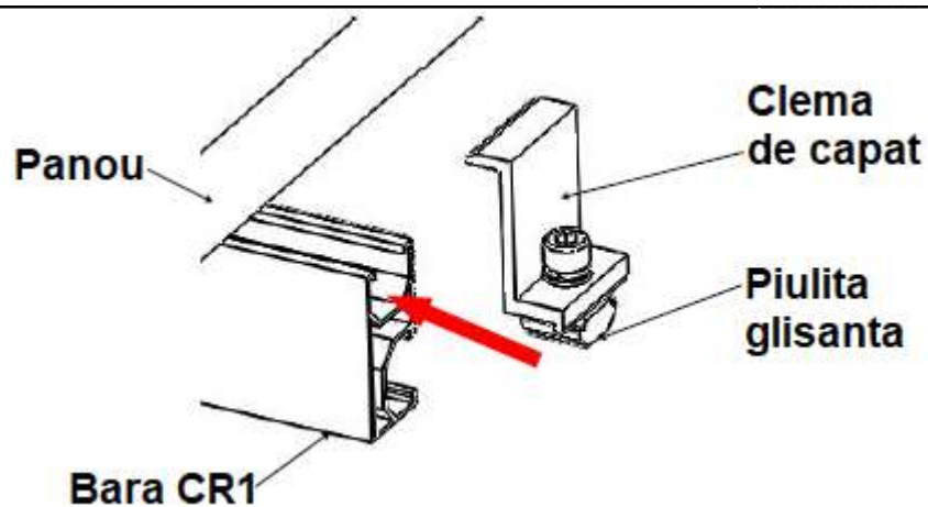
Fig. 3 - Instalare panou fotovoltaic - clema de capat
