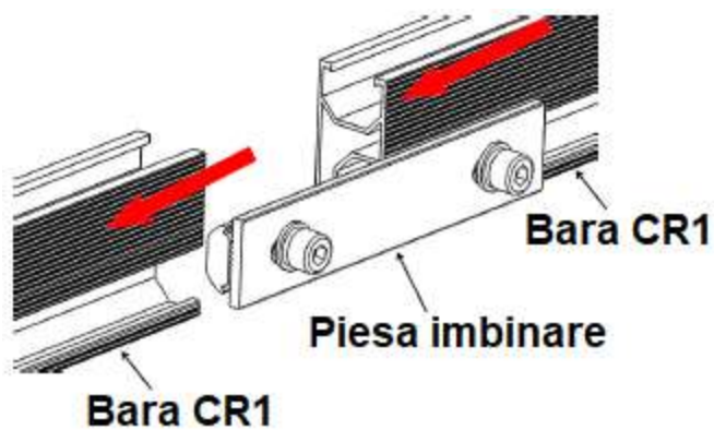
Fig. 5 - Imbinare bare CR1
