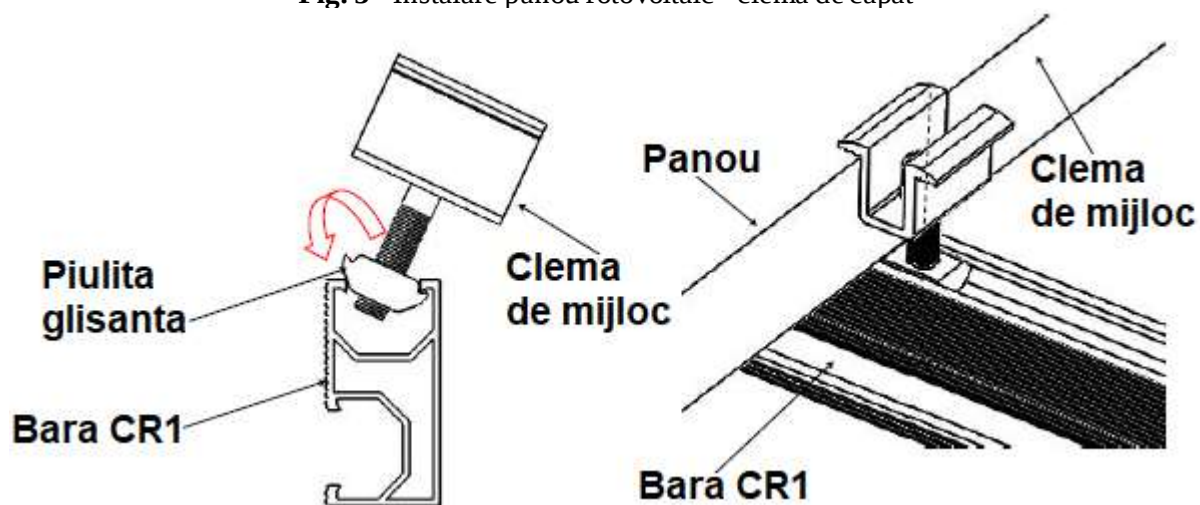
Fig. 4 - Instalare panou fotovoltaic - clema de mijloc
