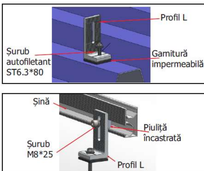
Fig. 2 - Clema L Feet - instalare
