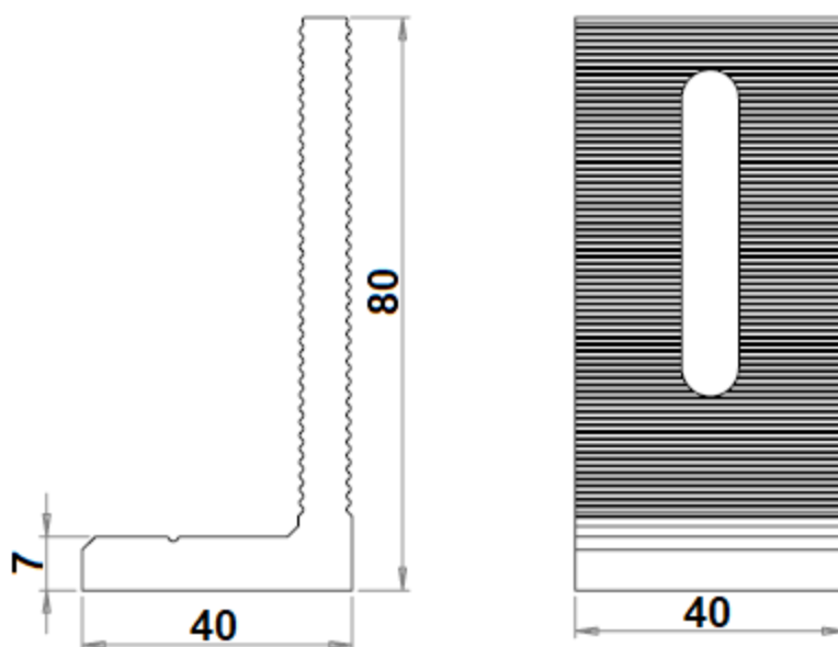
Fig. 1 - Clema L Feet – dimensiuni
