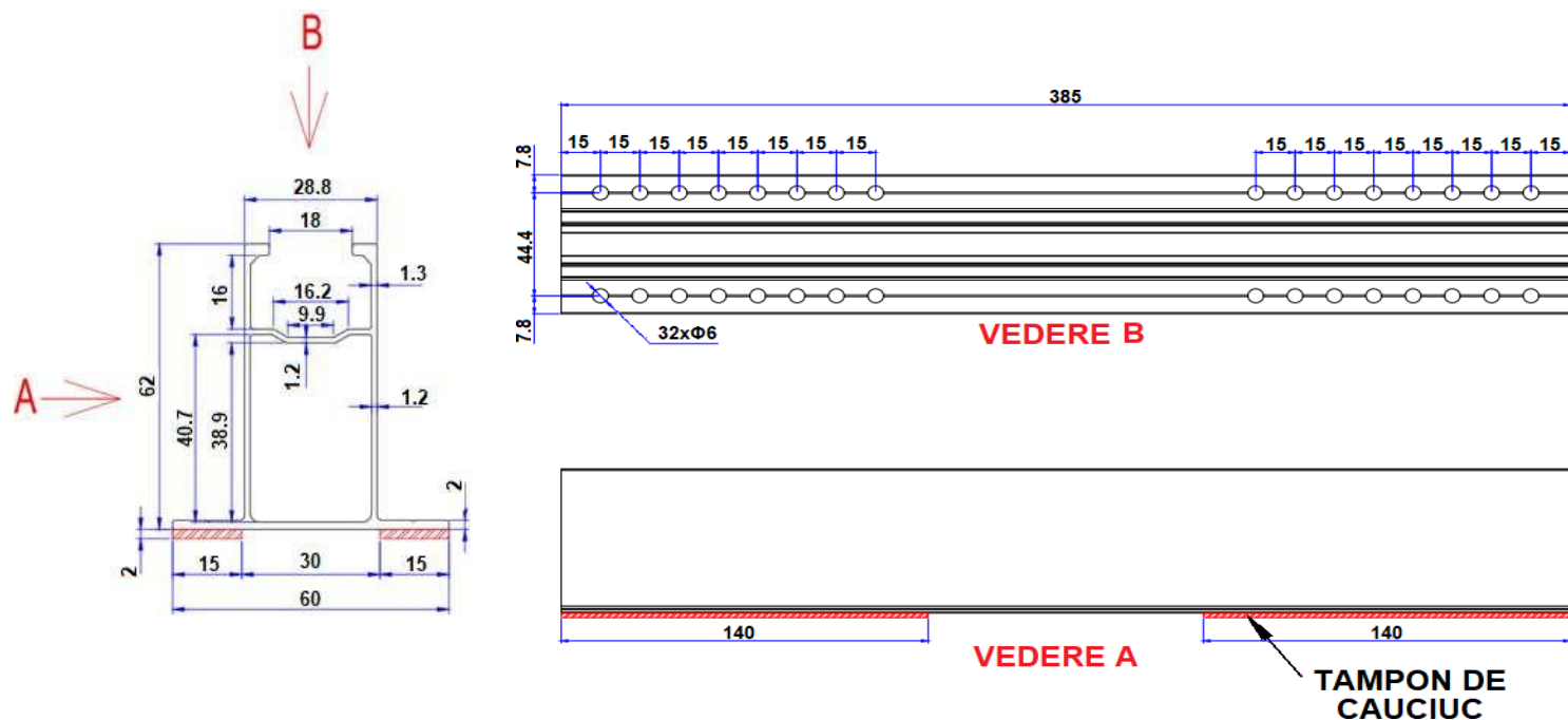
Fig. 1 - Sina mini rail H:62MM aluminiu sustinere panouri fotovoltaice - dimensiuni
