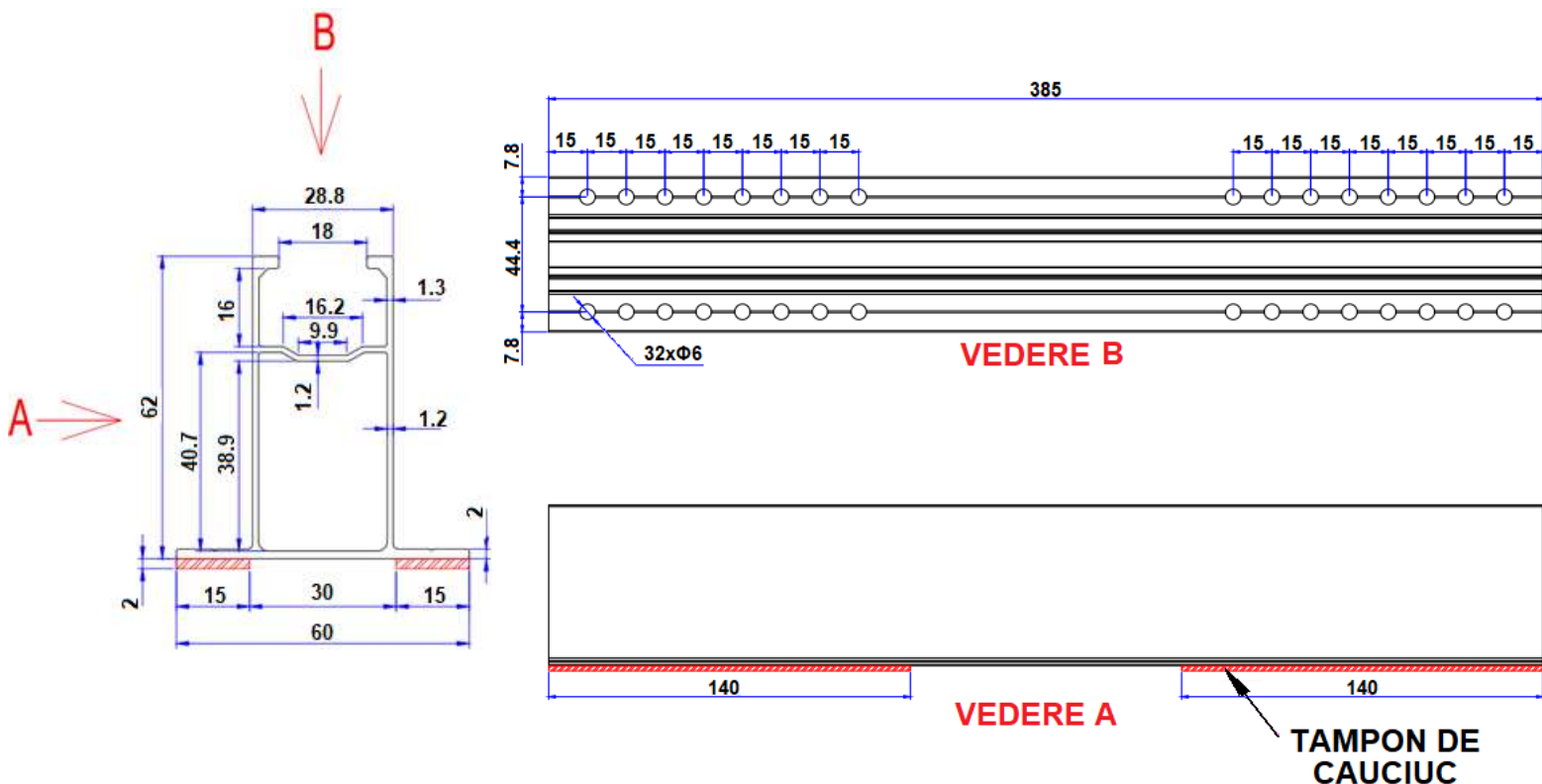
Fig. 1 - Sina mini rail H:62MM aluminiu sustinere panouri fotovoltaice - dimensiuni
