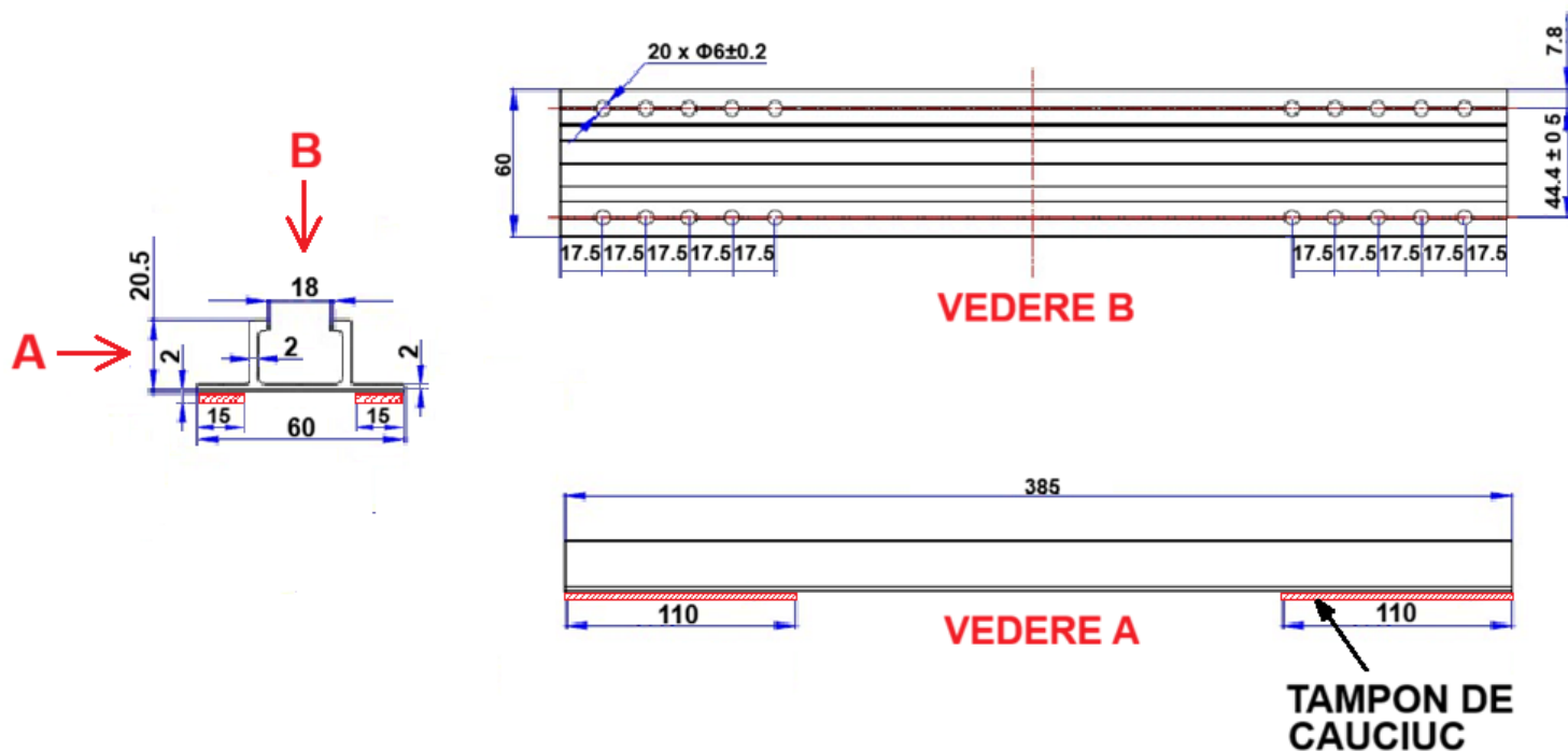
Fig. 1 – Sina mini rail aluminiu sustinere panouri fotovoltaice - dimensiuni
