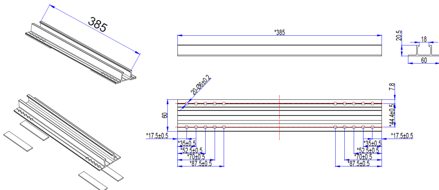
Fig. 1 - Sina mini rail aluminiu sustinere panouri fotovoltaice - dimensiuni
